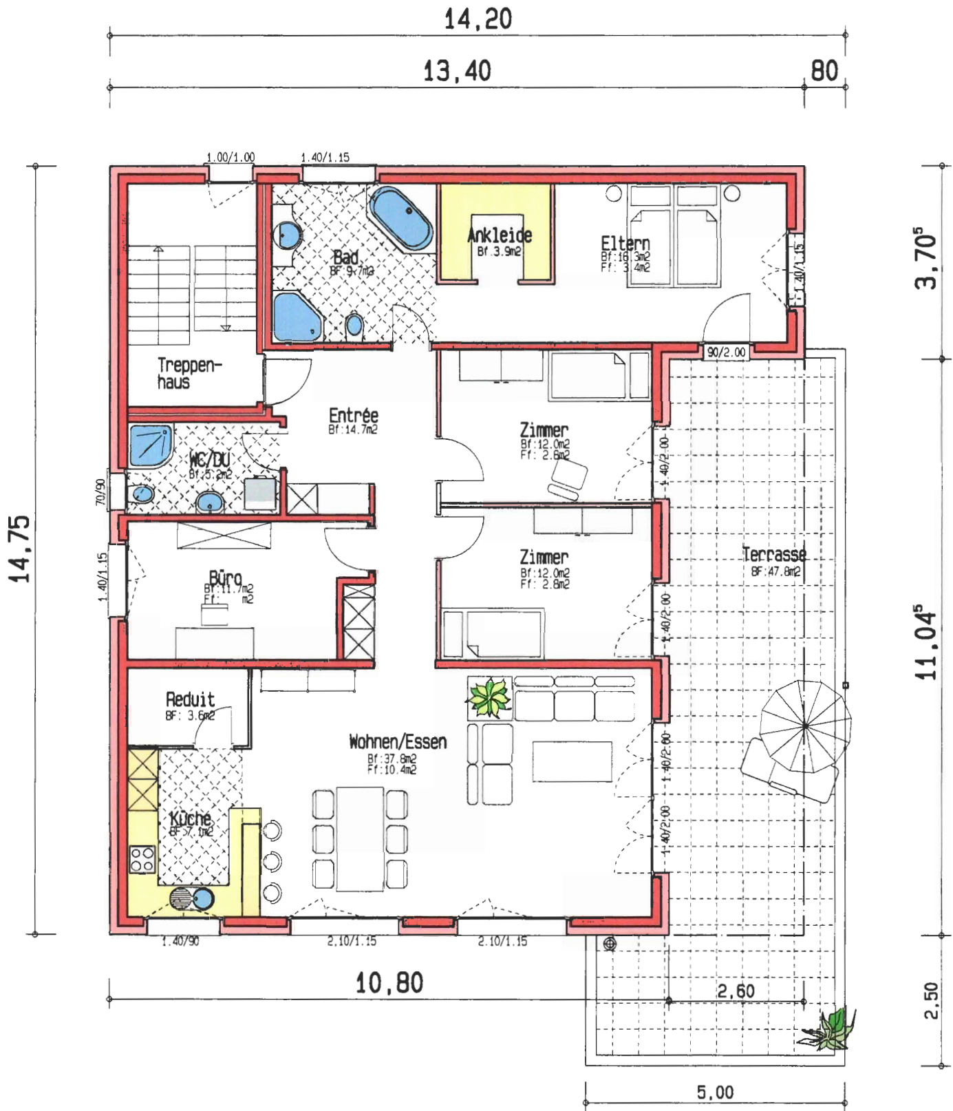
GRUNDRISS OBERGESCHOSS
