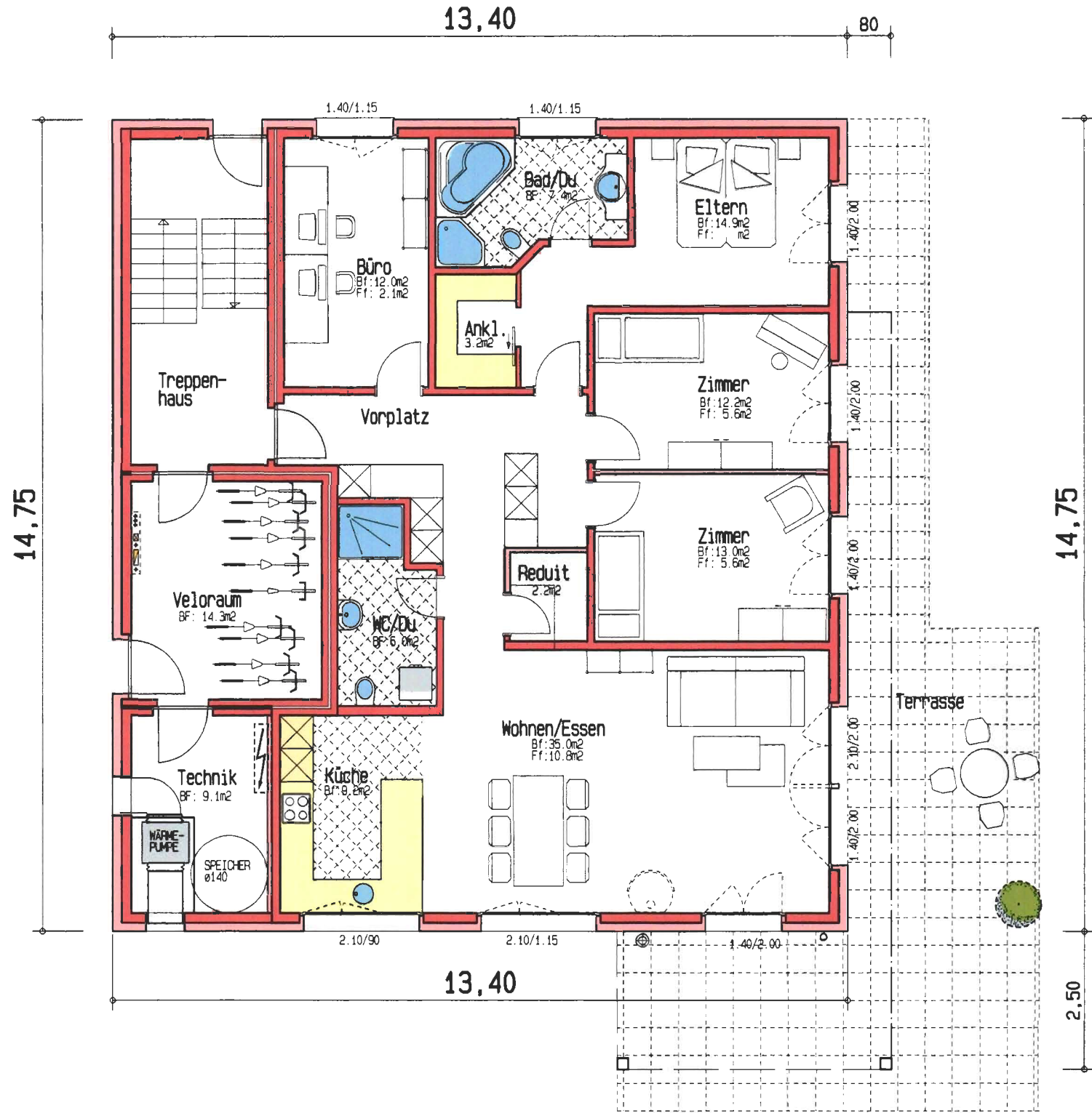
GRUNDRISS ERDGESCHOSS
