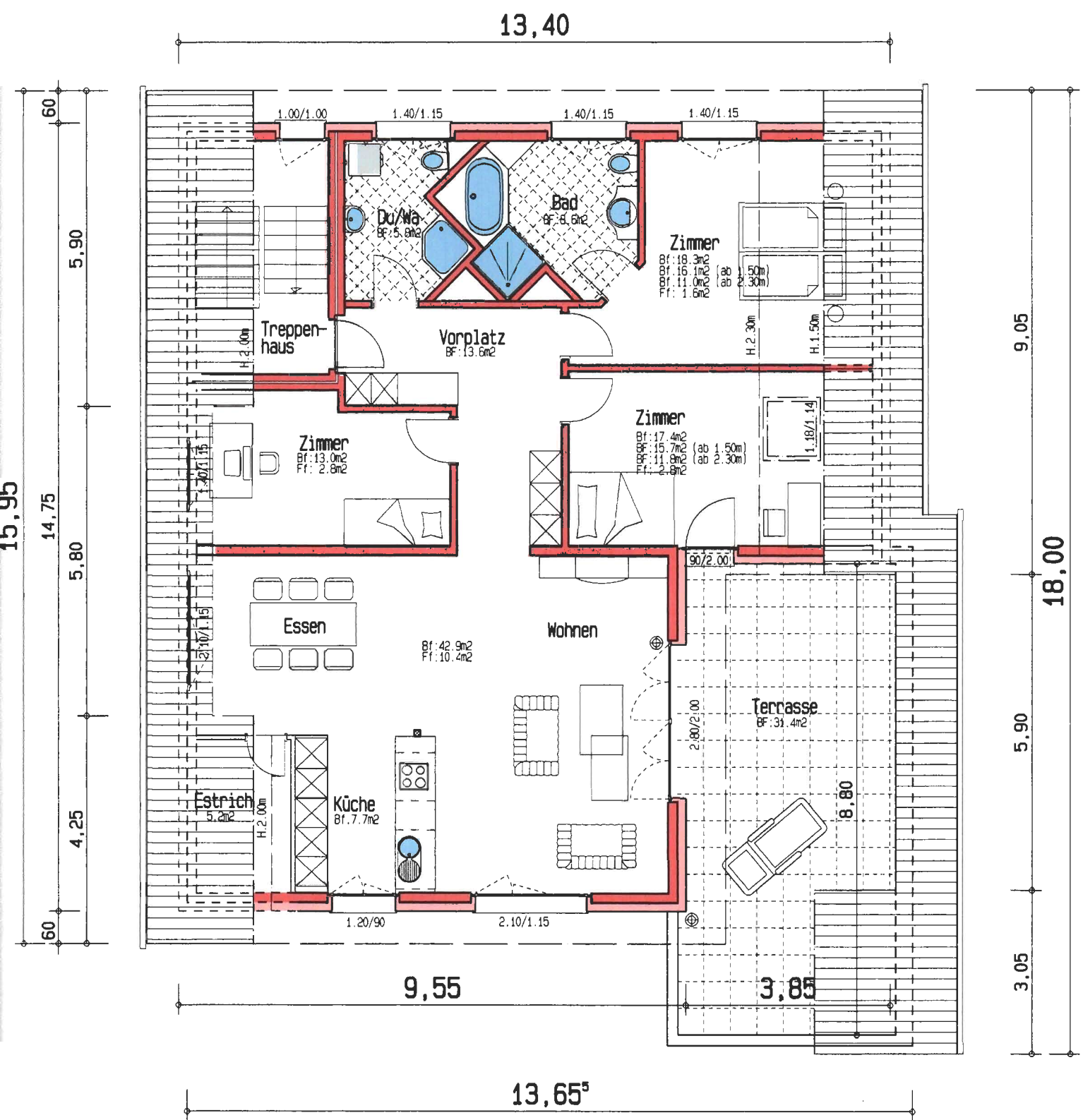
GRUNDRISS DACHGESCHOSS
